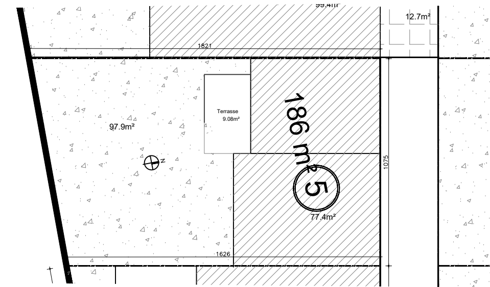
PLAN DE MASSE /Ech 1.200°
