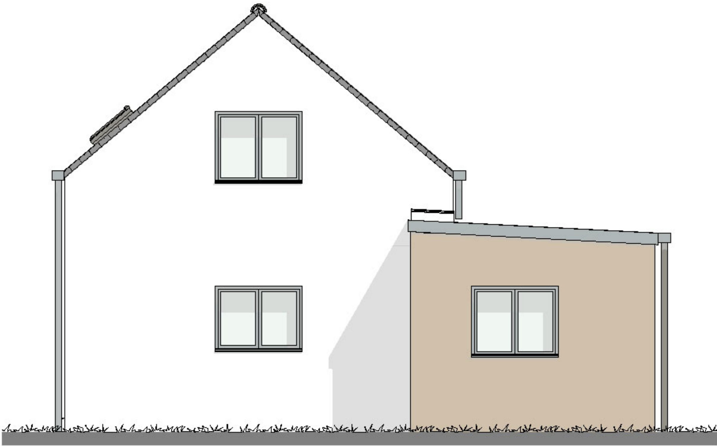
Façade nord
