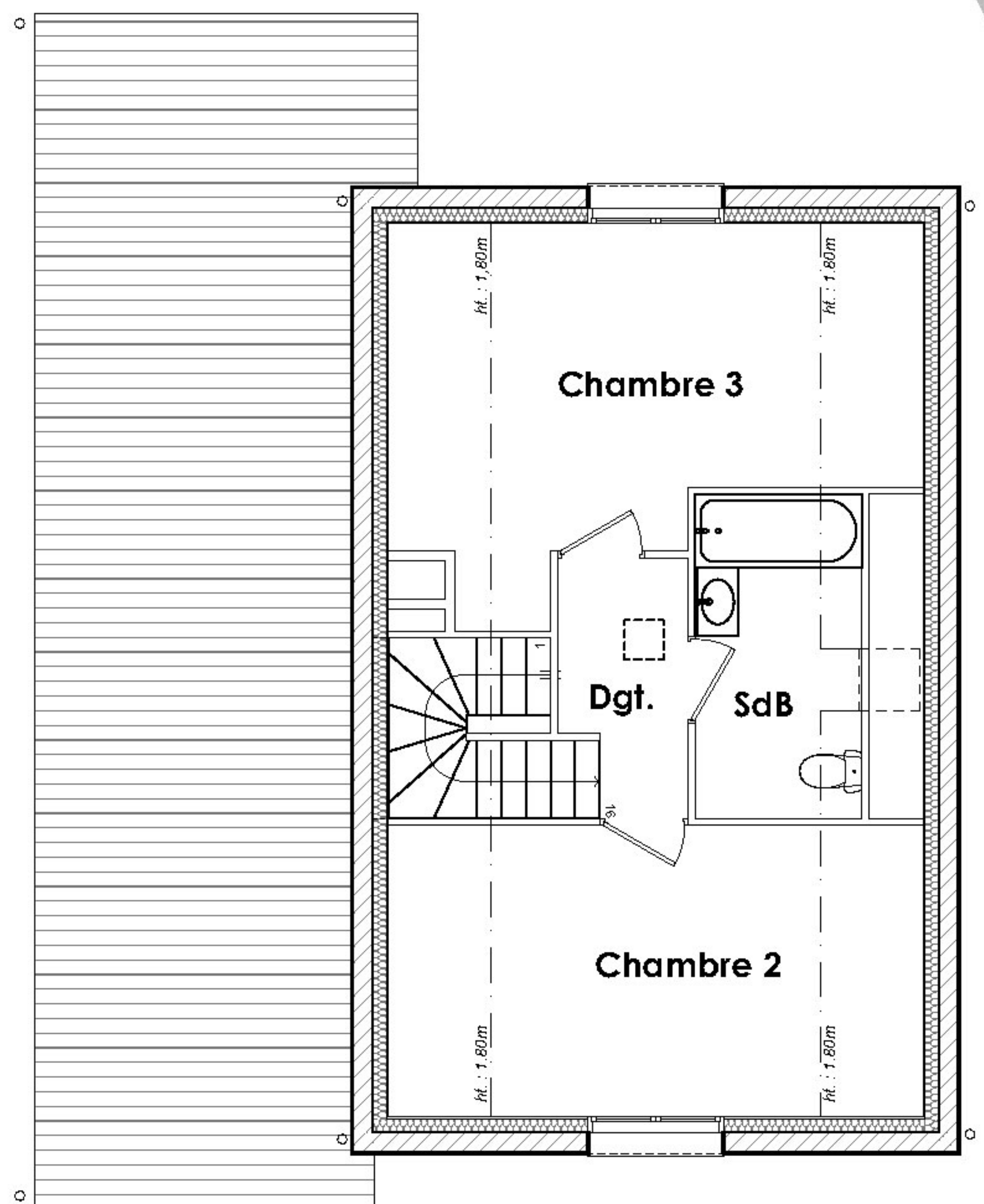
ETAGE
